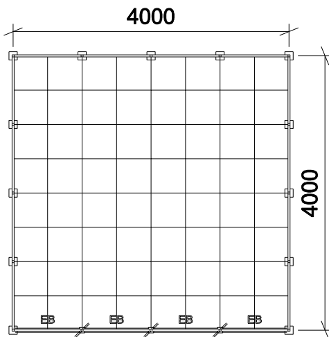
Grundriß:
